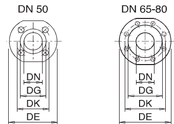
Flanges in accordance EN 1092-2 PN 25 - 40
